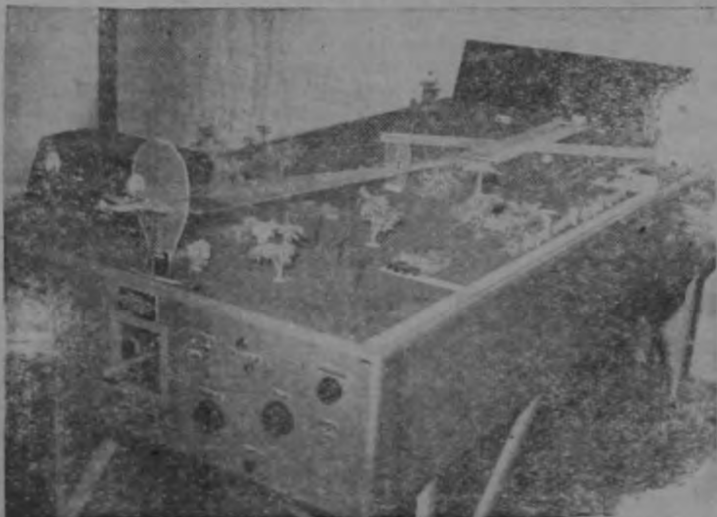
Modelo (de la administración de Aeronáutica Civil norteamericana) del sistema ILS y del control desde tierra (radar) para guiar las llegadas de los aviones. El aeroplano inclinado de plástico, representa el rayo electrónico de "guía"
